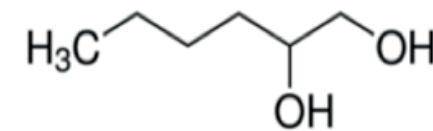
1, 2 - Hexanediol
